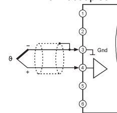
Thermocouples
